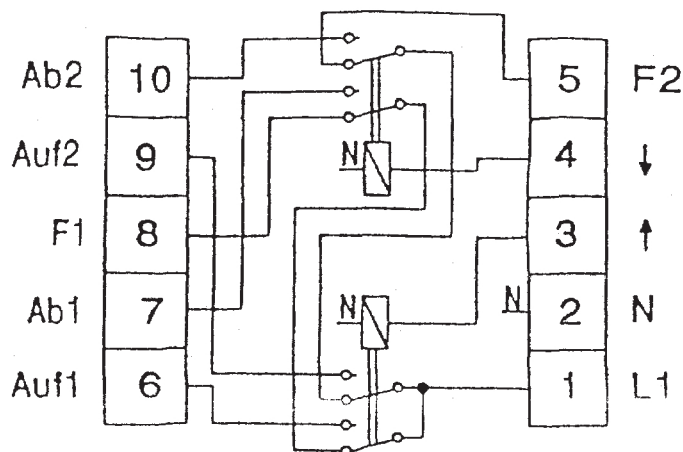
Innenschaltbild
